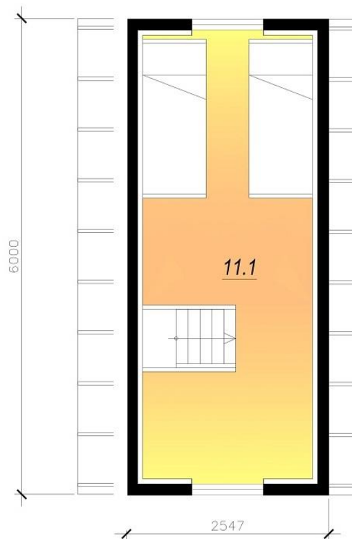
2 ЭТАЖ
